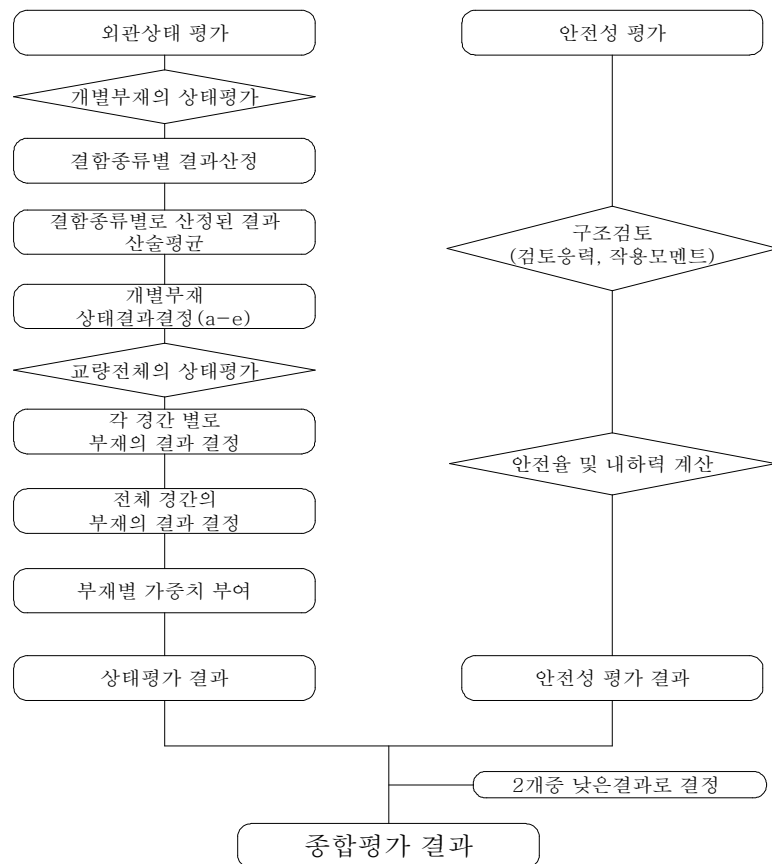
【그림 II-1.5.1】 종합평가 결과의 산정 흐름도
